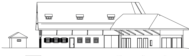
Ansicht Ost 1:500
