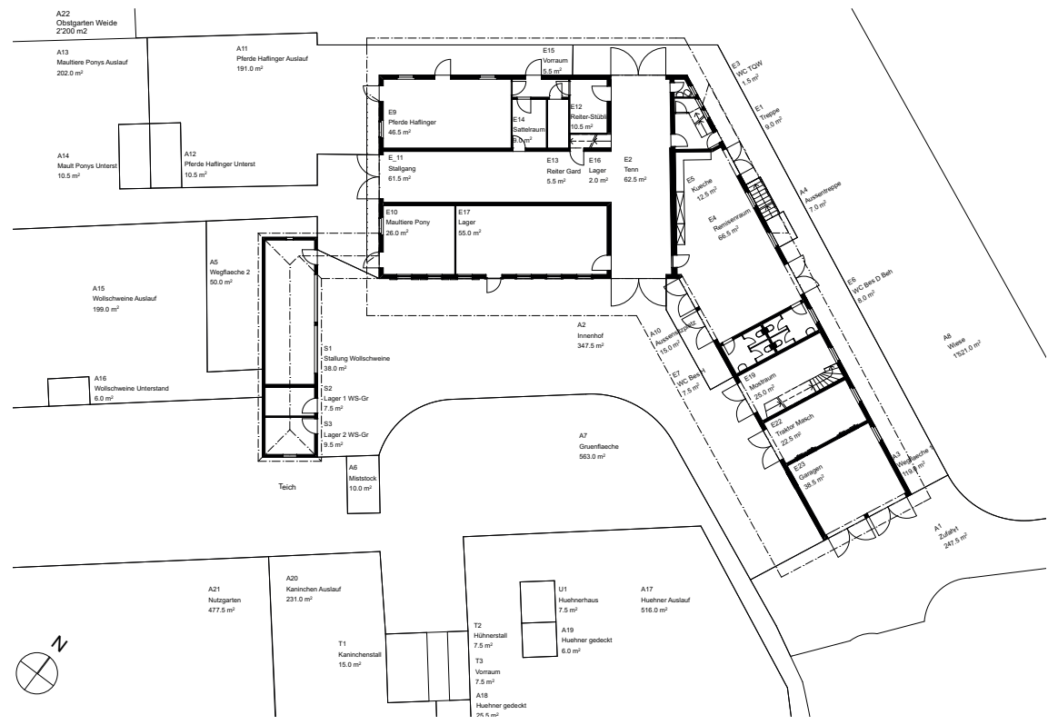
Erdgeschoss 1:500
